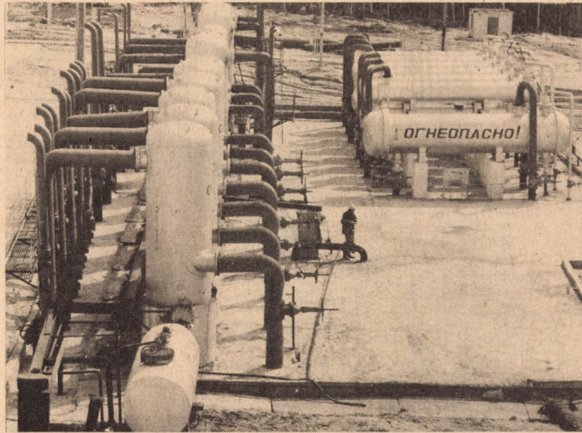
A SZIBÉRIAI OLAJVEZETÉK EGYIK RÉSZLETE
