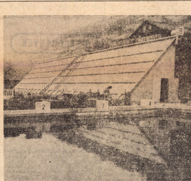
Most avatták fel az NDK-beli Freyburgban a világ első, napenergiával fűtött uszodáját: 240 elem gyűjti össze a nap sugarának hőjét, s egy csőrendszer segítségével fűtik az uszoda vizét
